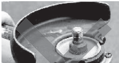
一般的な研削砥石用カバー
